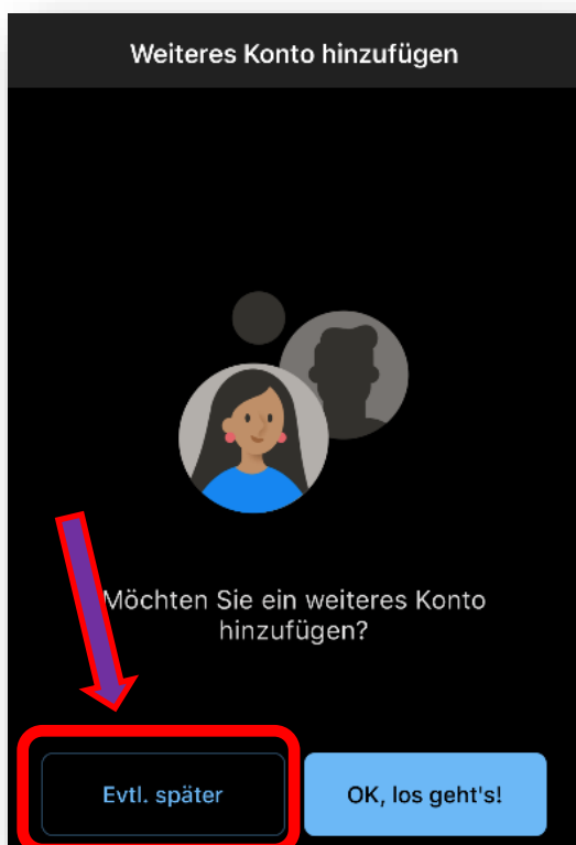
Abbildung 5: Einrichtung abgeschlossen
