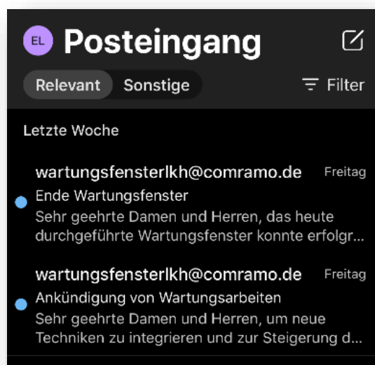
Abbildung 6: Ansicht Posteingang
